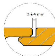
Tekening 10 Voldoende expansieruimte aanhouden tussen delen.
